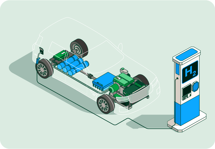
Vehículo eléctrico con pila de hidrógeno (FCEV)
