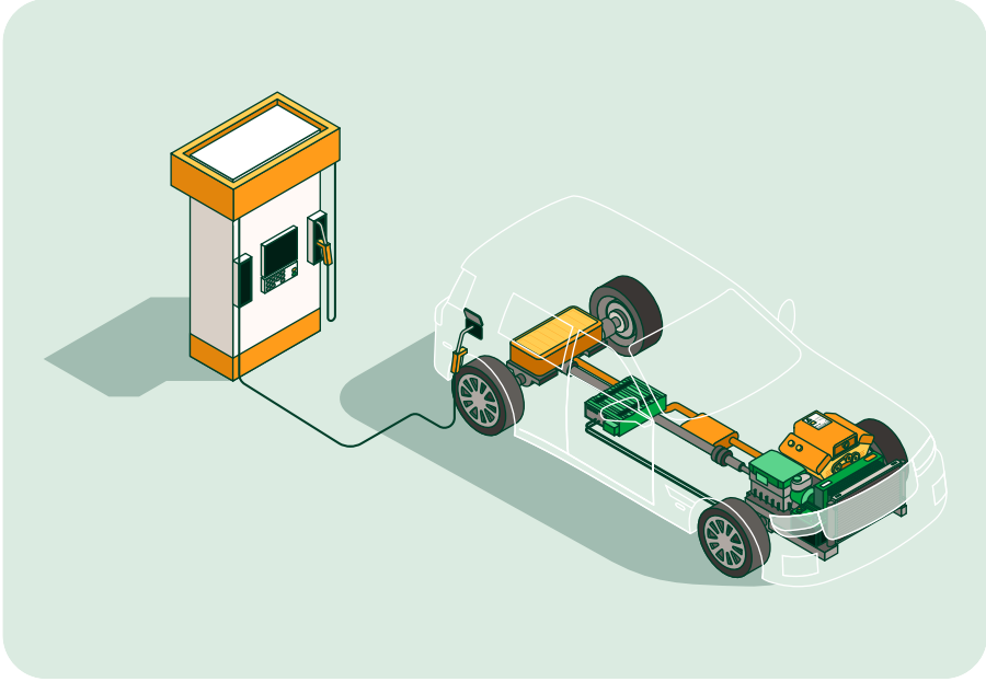
Veículo Híbrido (HEV)
