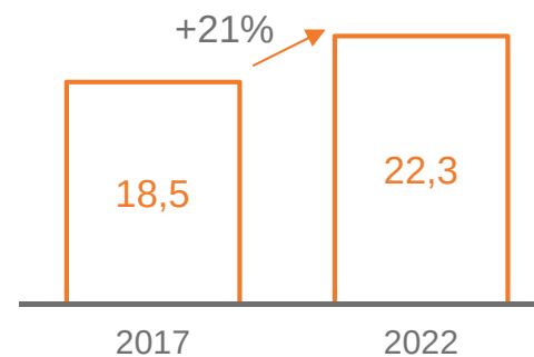
Producción (TWh)
