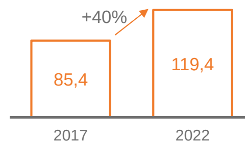
Producción (TWh)
